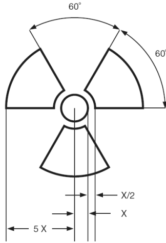
Hình 1. Dấu hiệu cảnh báo bức xạ. Bán kính tối thiểu X của đường tròn trung tâm là 4 (mm).
