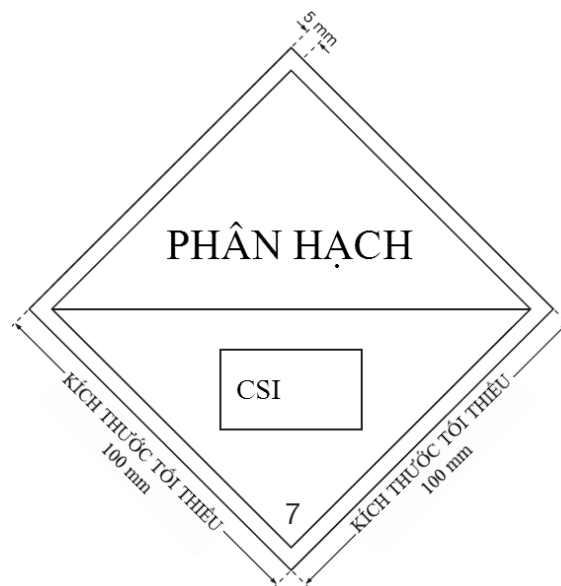
Hình 6. Nhãn chỉ số an toàn tối hạn: nền màu đen trắng, kích thước mỗi chiều tối thiểu 100 (mm).
