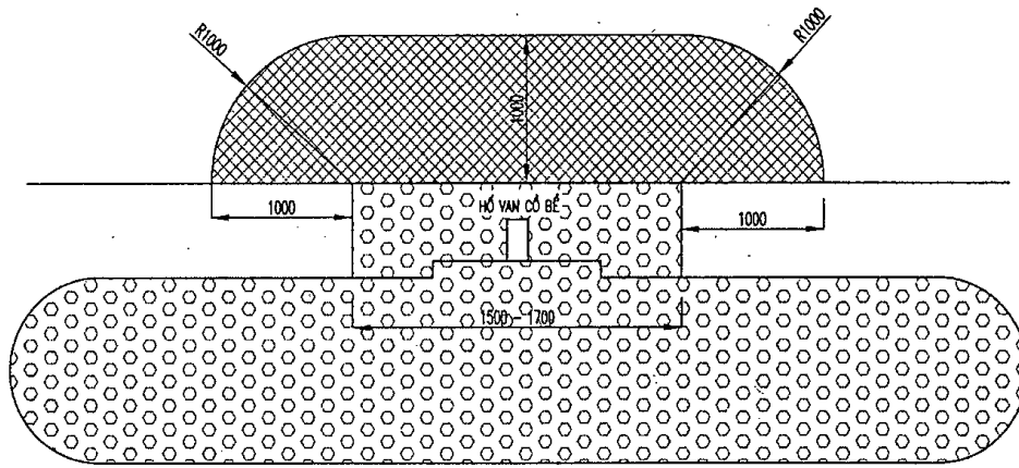
Hình 2: Vùng nguy hiểm cháy nổ bể chứa ngầm, họng nhập kín và họng thu hồi hơi ngay tại vị trí cỏ bể và đặt trong hố thao tác.
