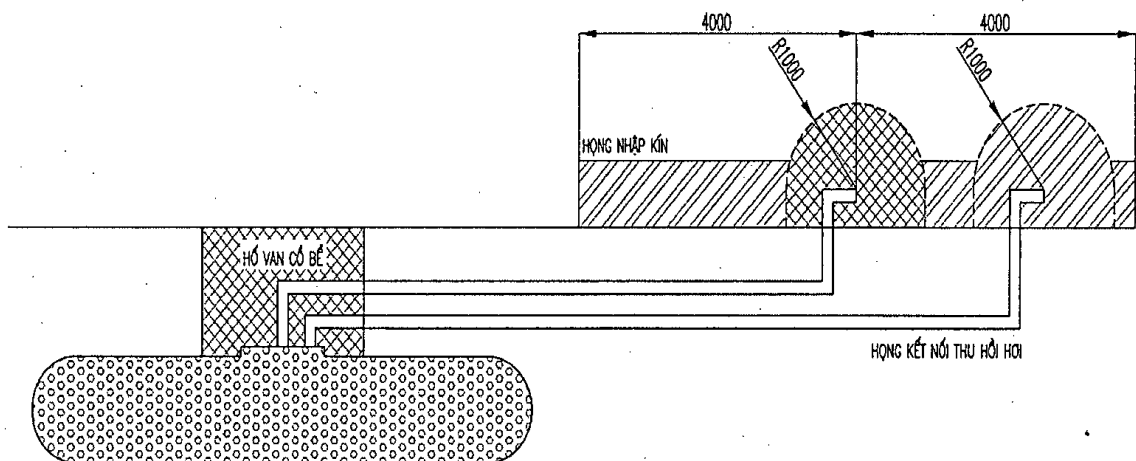
Hình 4: Vùng nguy hiểm cháy nổ bể chứa ngầm, họng nhập kín và họng thu hồi hơi xa vị trí cỏ bể và không đặt trong hố thao tác.
