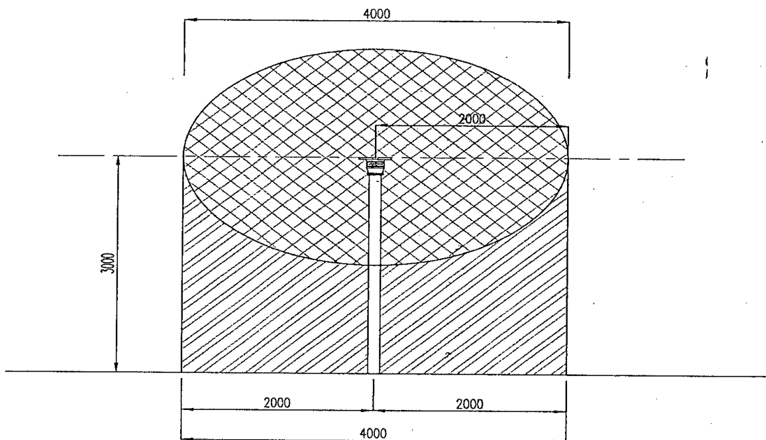
Hình 6: Vùng nguy hiểm cháy nổ của van thử khi không có thu hồi hơi.
