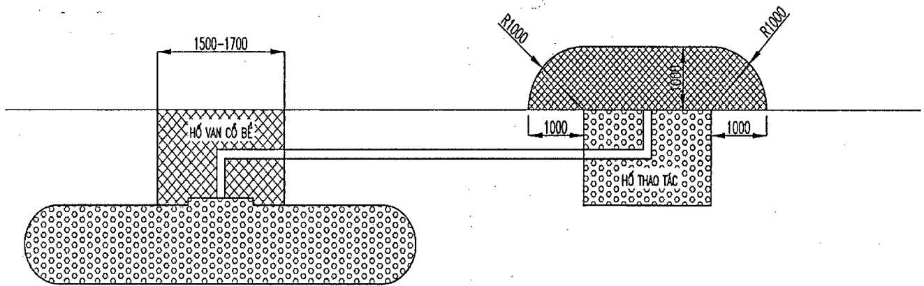
Hình 3: Vùng nguy hiểm cháy nổ bể chứa ngầm, họng nhập kín và họng thu hồi hơi xa vị trí cỏ bể và đặt trong hố thao tác.
