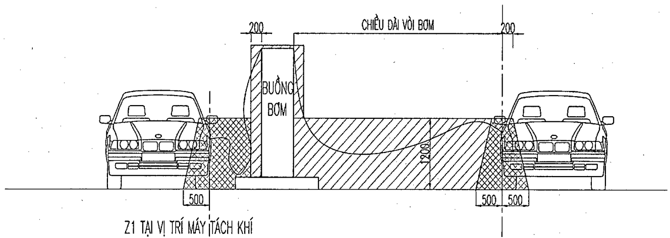
Hình 8: Vùng nguy hiểm cháy nổ xung quanh vị trí cột bơm khi đan bán hàng cho phương tiện giao thông.
