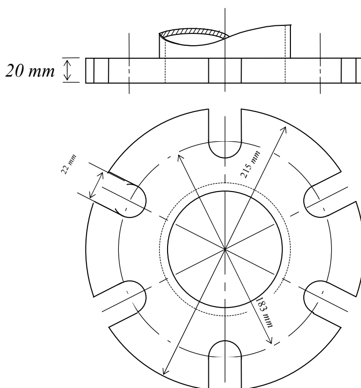
Hình 1. Bích nối xả tiêu chuẩn
