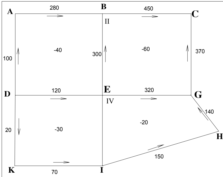
Hình 2. Gia số trường \Delta T của tuyến chuẩn đo 2 lần độc lập
