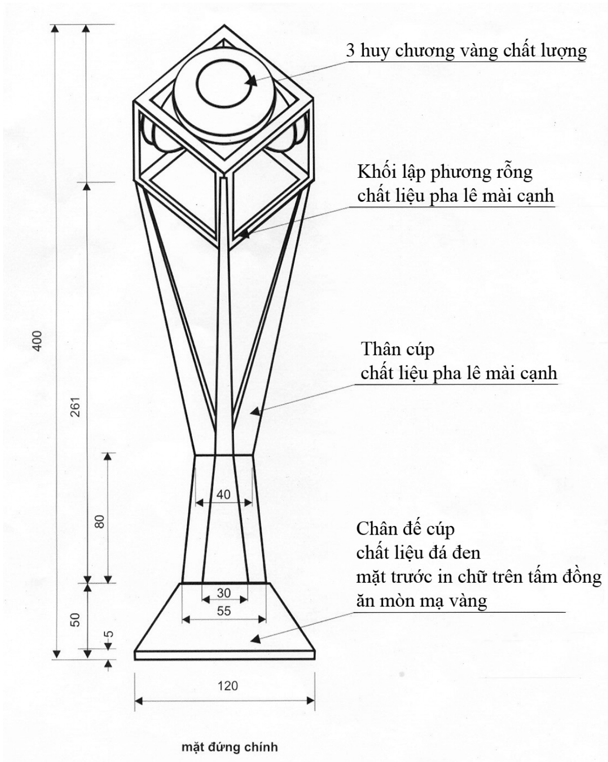
Hình 2. Kích thước mặt trước của Cúp Giải thưởng Quốc gia về chất lượng công trình xây dựng
