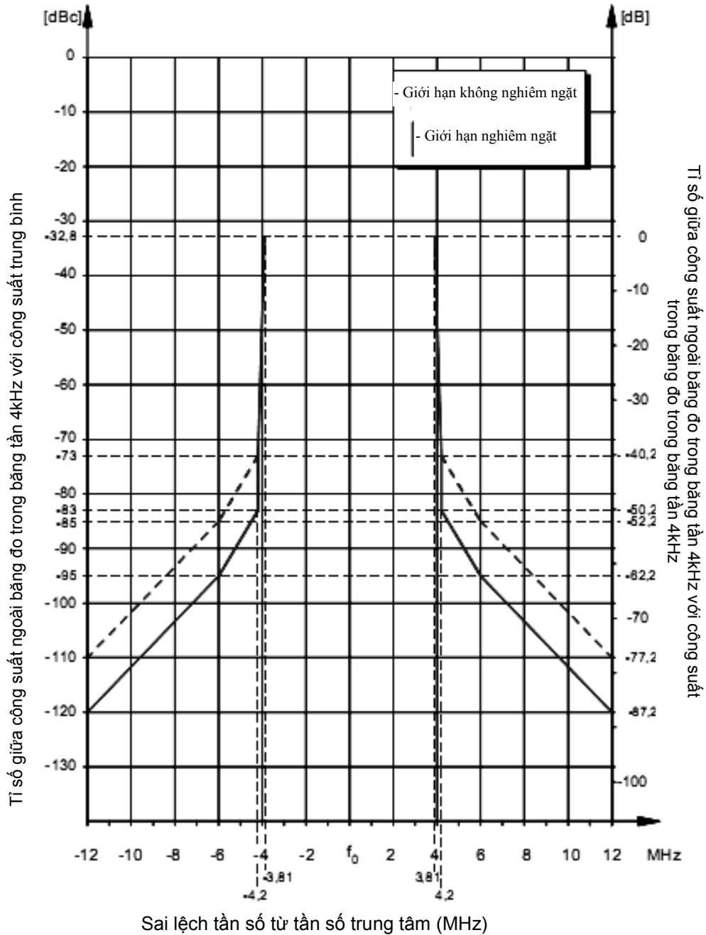
Hình 4. Giới hạn phát xạ ngoài băng đối với các máy phát DVB-T2 có công suất từ 25W trở lên
