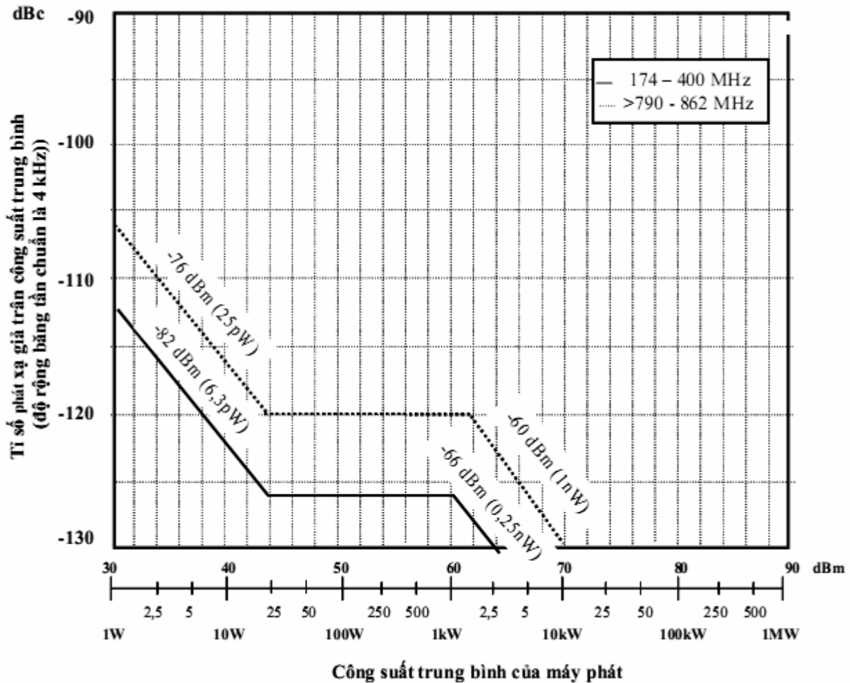
Hình 3. Các giới hạn phát xạ giả đối với máy phát DVB-T2 (độ rộng băng tần chuẩn là 4 kHz)
