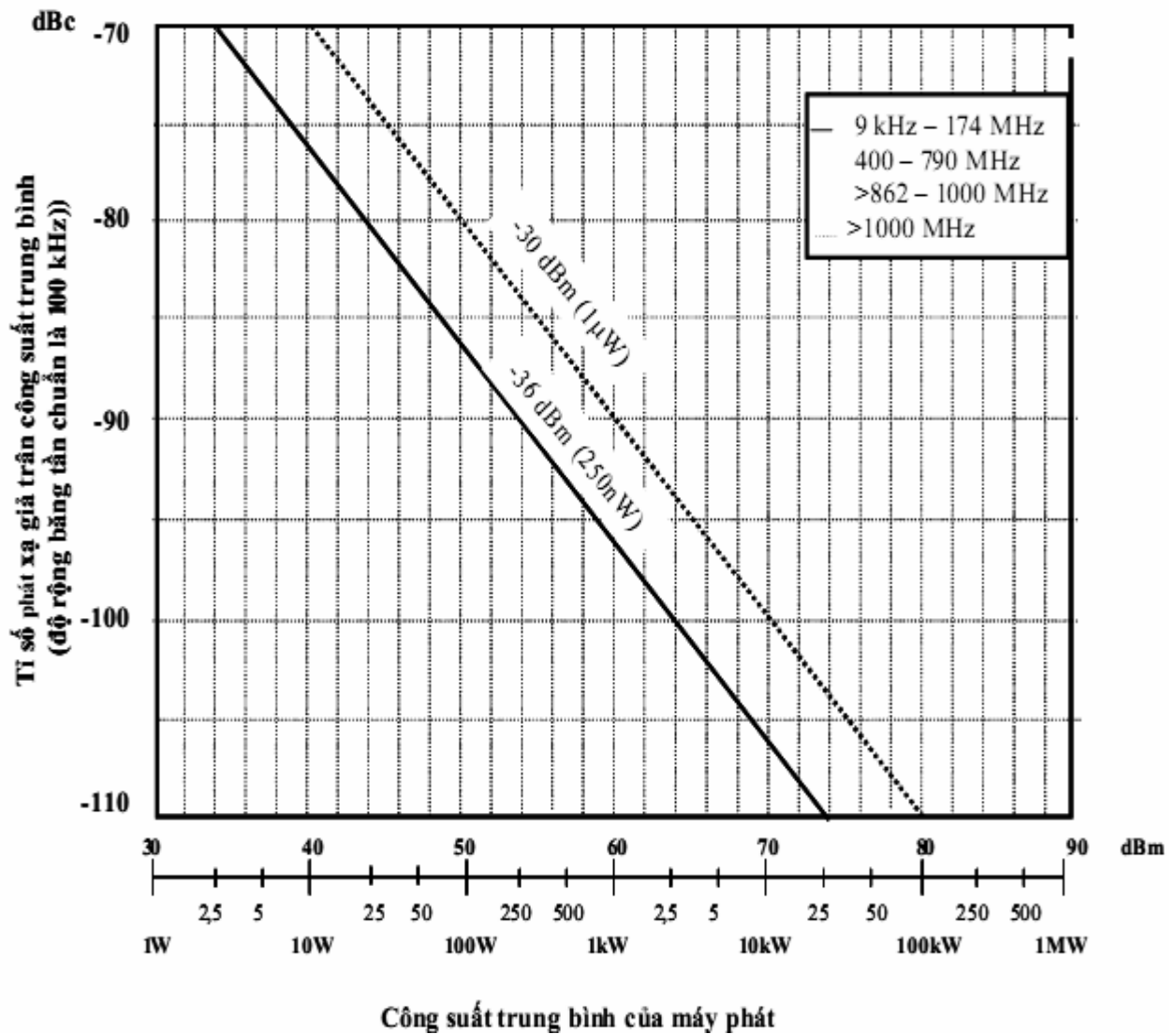
Hình 2. Các giới hạn phát xạ giả đối với máy phát DVB-T2 (độ rộng băng tần chuẩn là 100 kHz)
